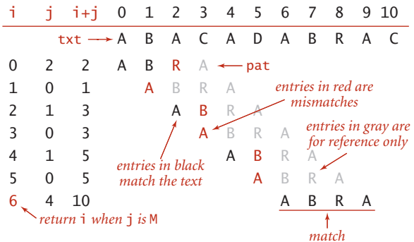
Brute-force substring search
